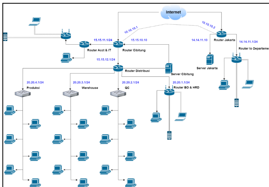
Gambar 01 : Topologi Jaringan PT Indofood CBP Sukses Makmur Tbk
