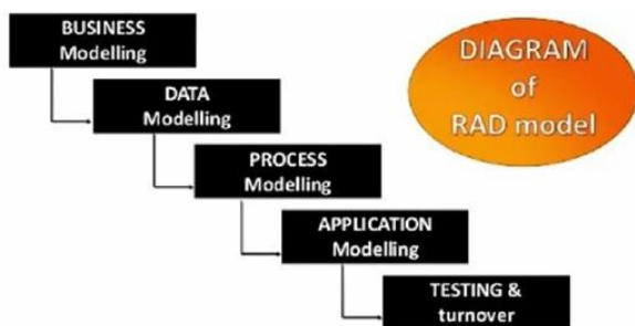
Gambar 1 Metode RAD
